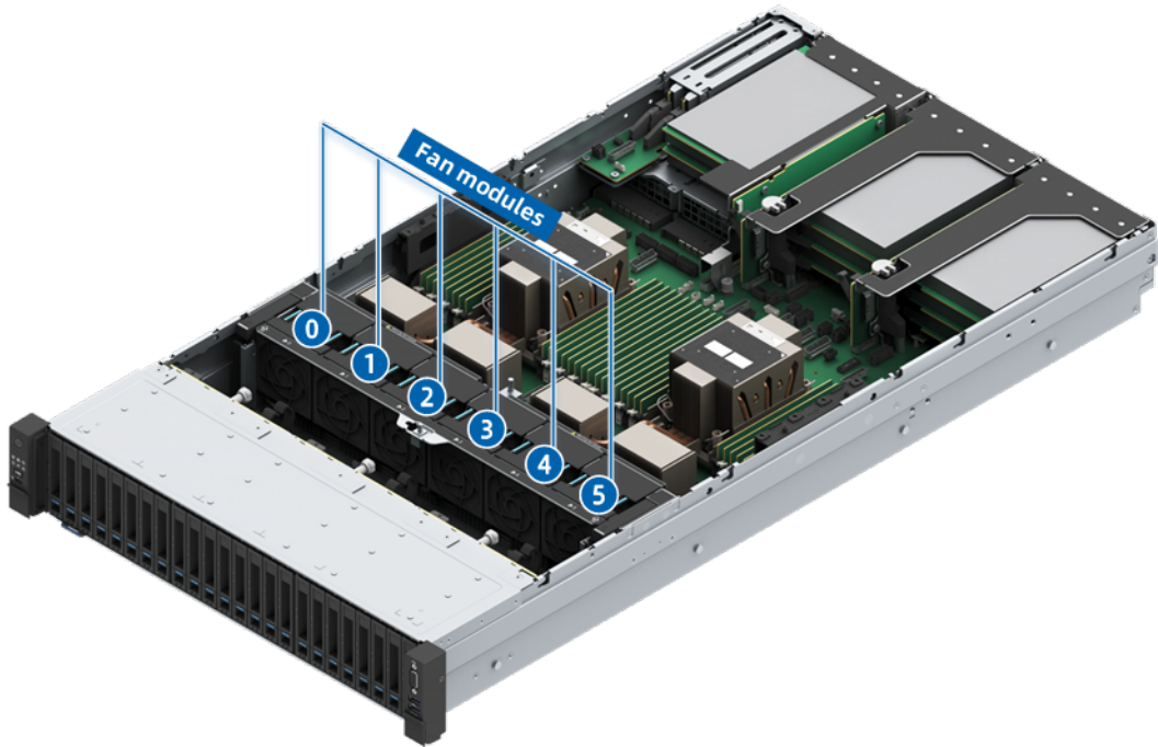
图 5-25 风扇模组的位置
