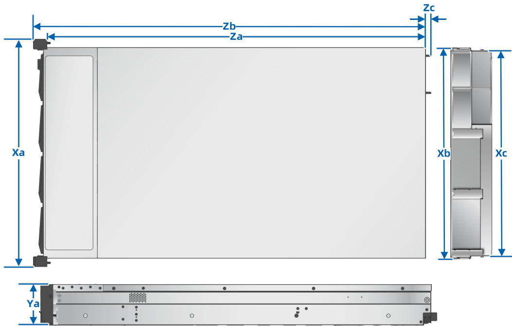
图 6-1 主机尺寸
