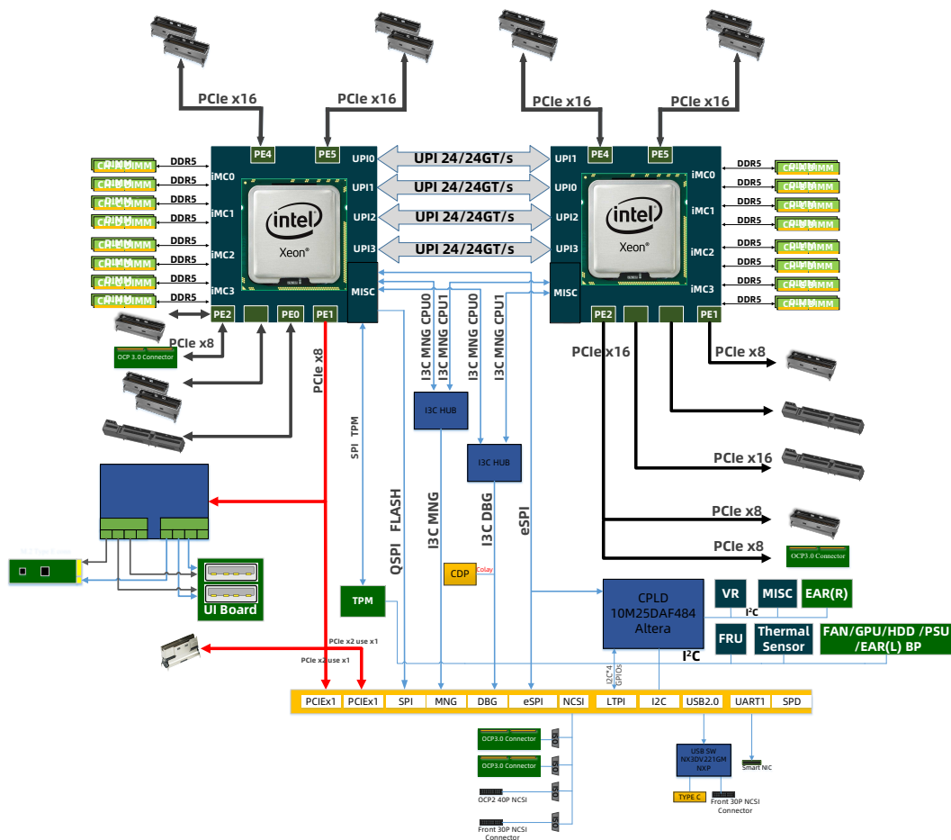
图 4-1 RS5220G6系列逻辑结构
