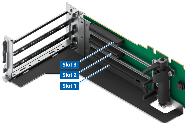
图 5-17 PCIe 转接卡模组 0 (1 个 x16 插槽 + 2 个 x8 插槽)
