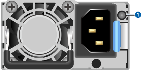
图 5-24 电源指示灯说明
