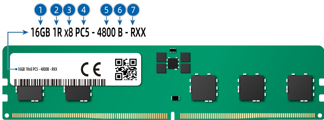
图 5-7 内存标识
