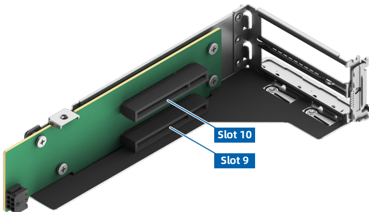
图 5-22 PCIe 转接卡模组 4 (2 个 x8 插槽)
