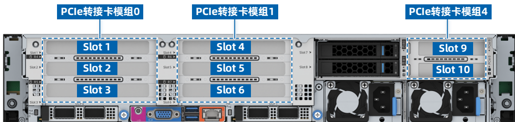
图 5-15 PCIe 插槽-8 张 PCIe 扩展卡后窗
