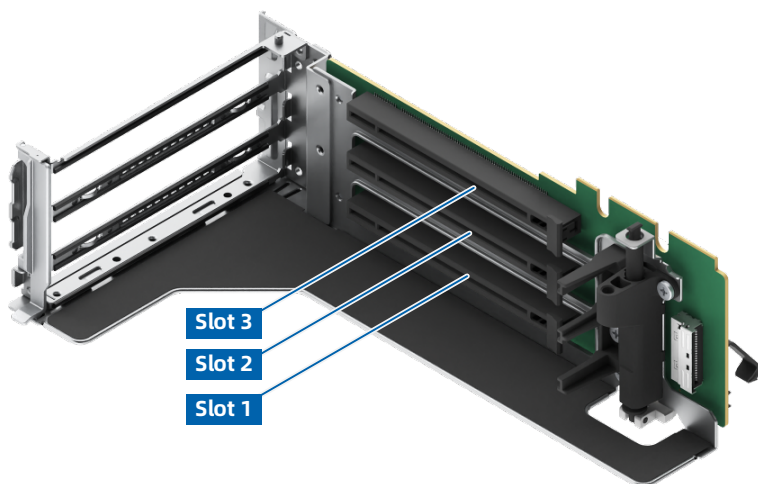
图 5-16 PCIe 转接卡模组 0 (3 个 x16 插槽)
