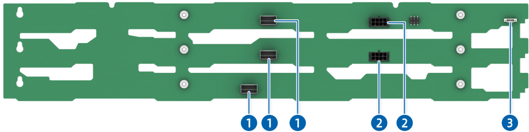
图 5-31 12 × 3.5 英寸硬盘配置 (12 × SAS/SATA) 背板
