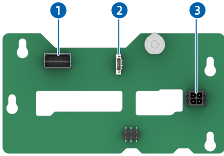
图 5-34 2 × 3.5 英寸硬盘配置 (2 × SAS/SATA) 背板
