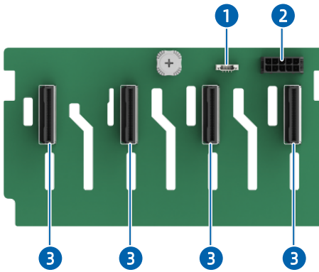
图 5-33 8 × E3.S 硬盘配置背板
