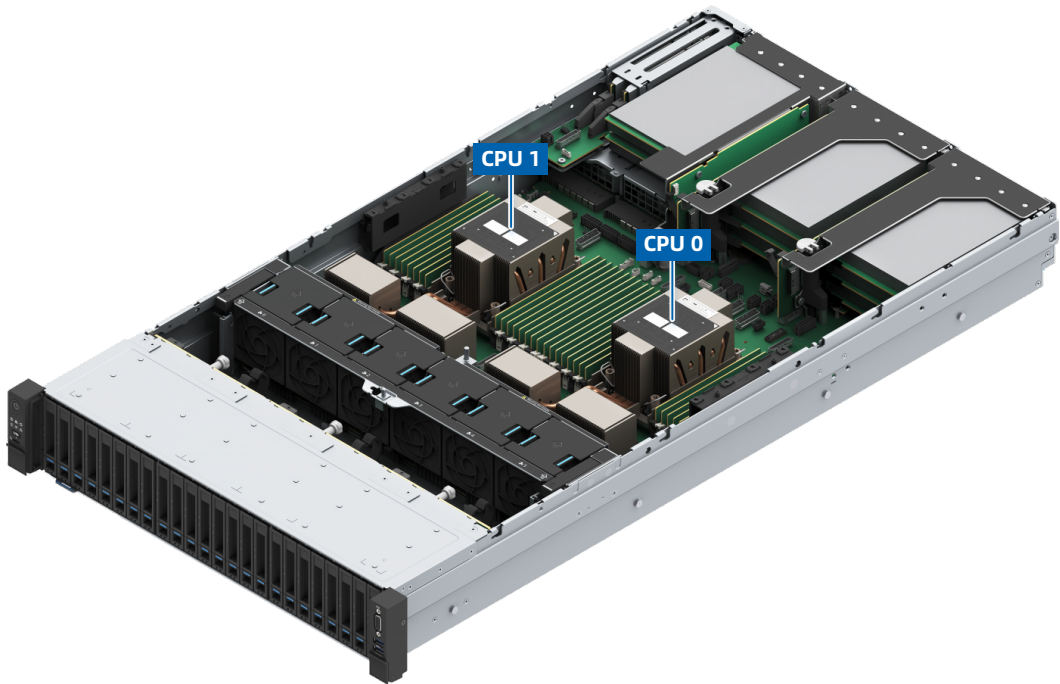
图 5-6 处理器位置
