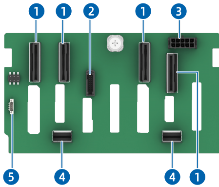
图 5-32 8 × 2.5 英寸硬盘配置 (8 × SAS/SATA/NVMe) 背板
