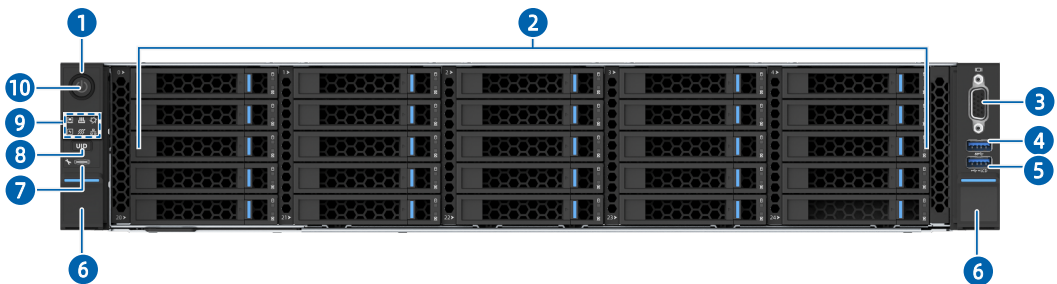
图 5-3 前面板外观
