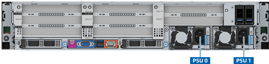
图 5-23 电源模块位置
