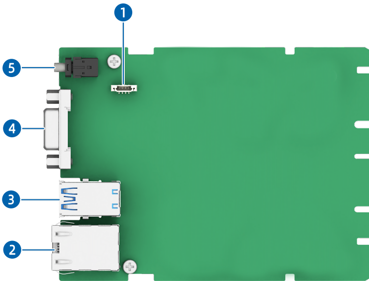
图 5-37 DC-SCM 板
