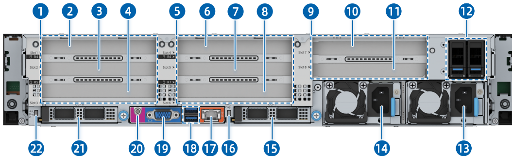
图 5-4 后面板外观
