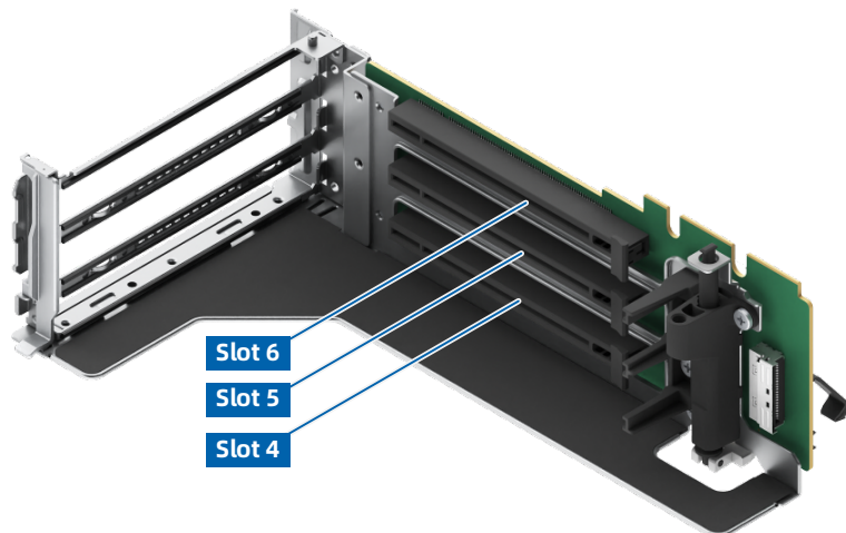
图 5-18 PCIe 转接卡模组 1 (3 个 x16 插槽)
