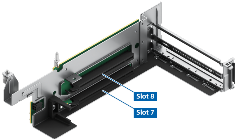
图 5-20 PCIe 转接卡模组 2 (2 个 x16 插槽)
