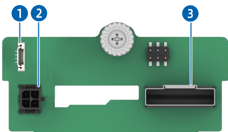
图 5-36 2 × 2.5 英寸硬盘配置 (2 × NVMe) 背板
