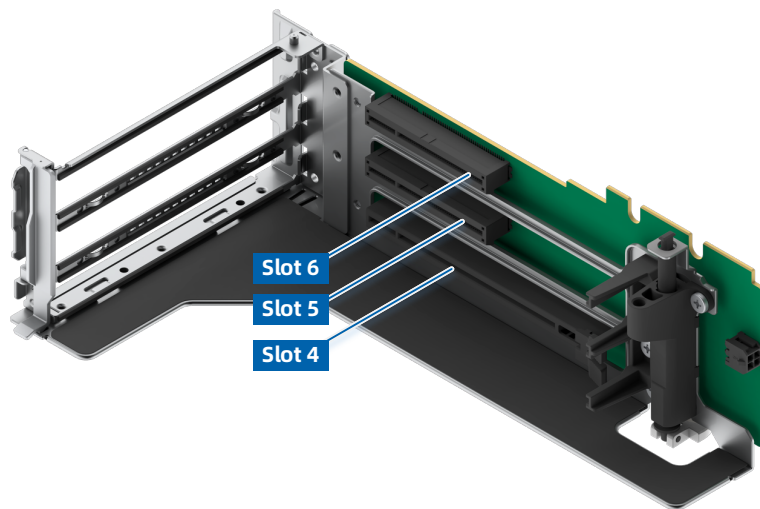
图 5-19 PCIe 转接卡模组 1 (1 个 x16 插槽 + 2 个 x8 插槽)
