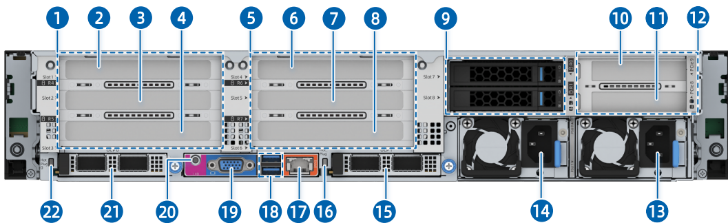
图 5-5 后面板外观
