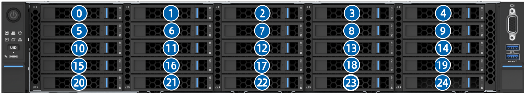
图 5-11 硬盘编号
