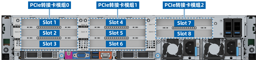
图 5-14 PCIe 插槽-8 张 PCIe 扩展卡后窗
