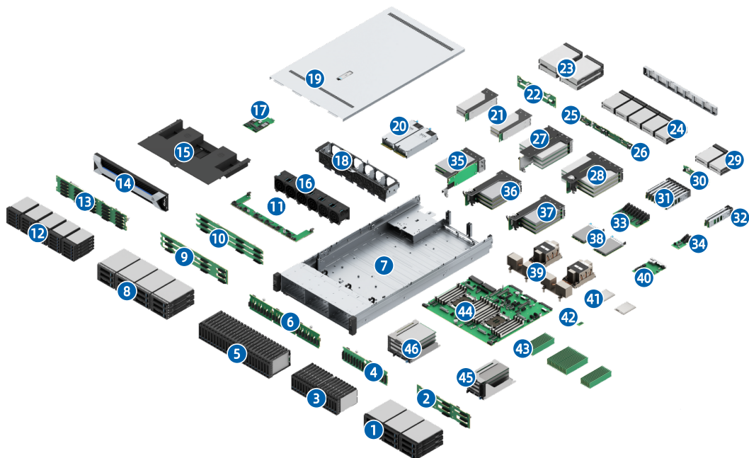
图 3-1 物理结构
