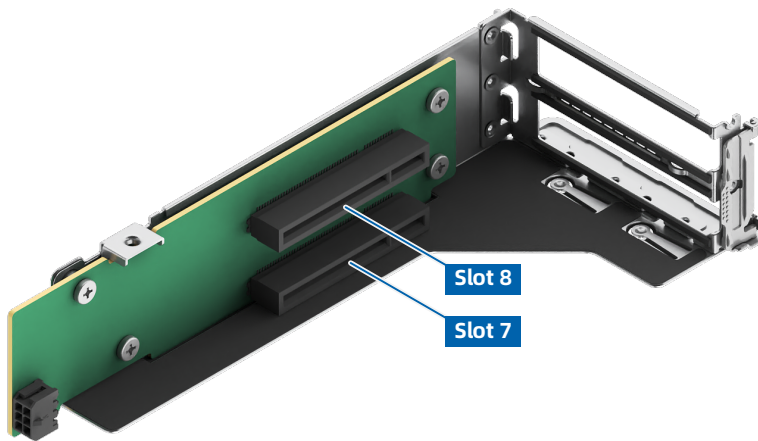
图 5-21 PCIe 转接卡模组 3 (2 个 x8 插槽)
