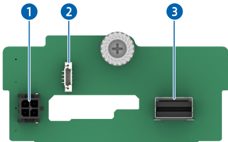
图 5-35 2 × 2.5 英寸硬盘配置 (2 × SAS/SATA) 背板
